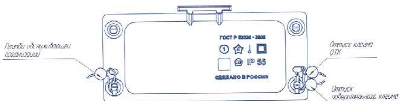
Рисунок 2 – Схема пломбирования счётчика
